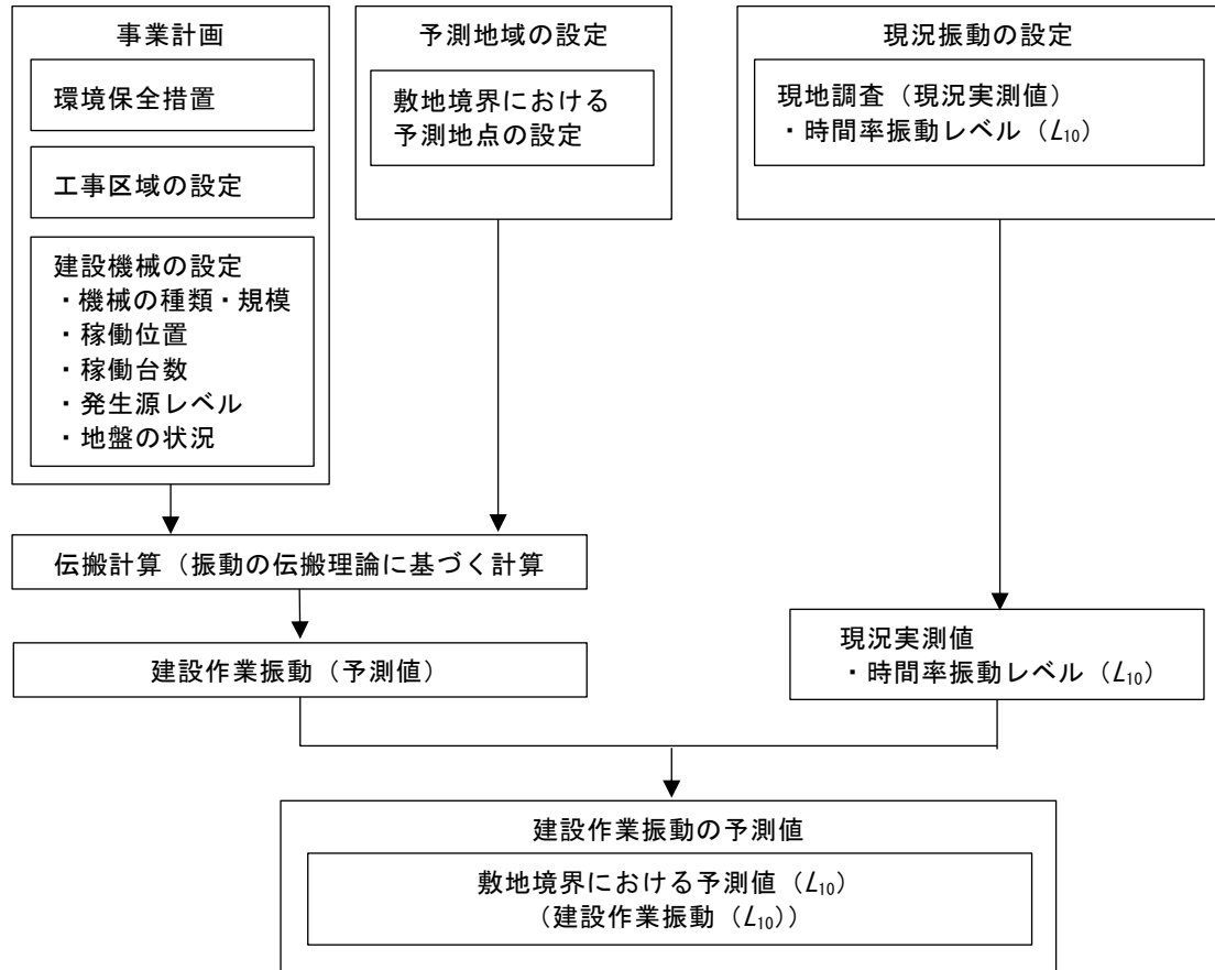
図 12. 1. 1. 3-4 建設機械の稼働に伴う振動の予測手順
