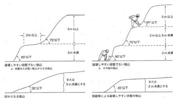
図1 掘削面の勾配
